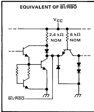
'46A, '47A, '48
