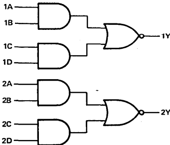
'L51, 'LS51
