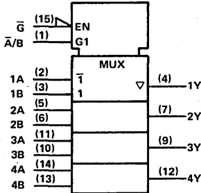
'S257
