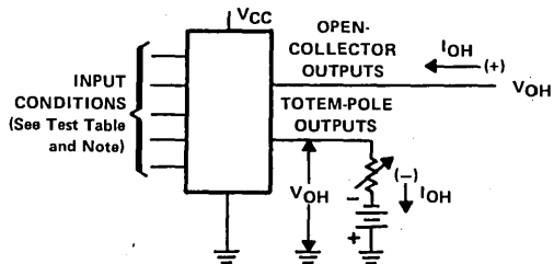
FIGURE 1. V_{IH} , V_{IL} , V_{OH} , I_{OH}
