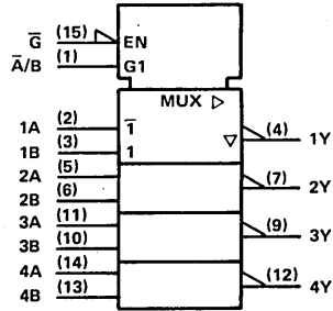
'S258
