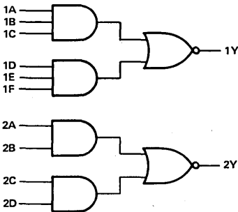
'L51, 'LS51
