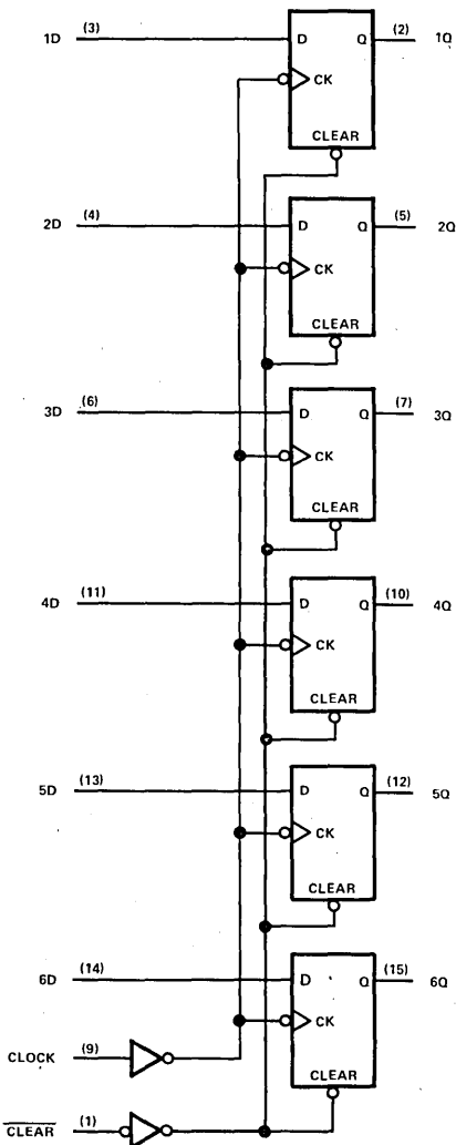
'174, 'LS174, 'S174
