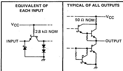
'S283
