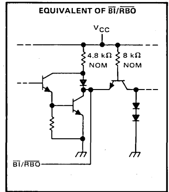
'L46, 'L47
