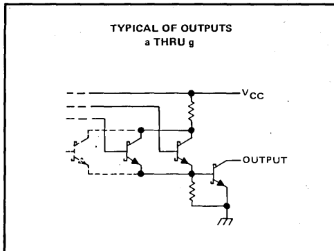
'LS249
