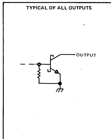
'LS170
