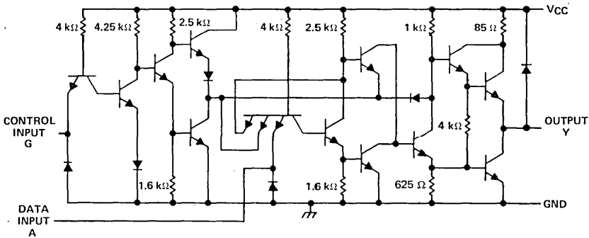
'126 CIRCUITS
