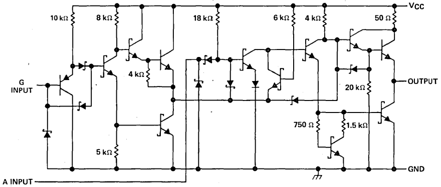
'LS125A CIRCUITS
