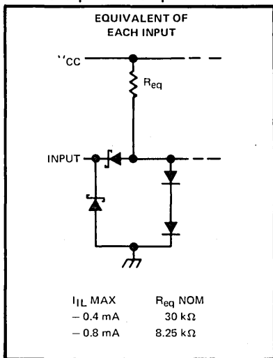
'LS113A
