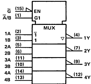
'S258
