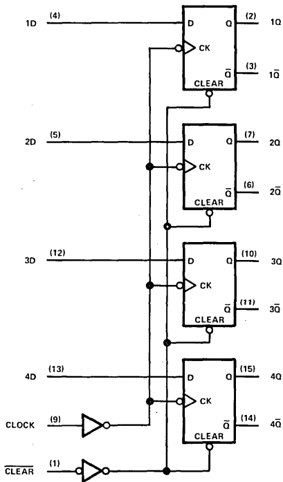
'175, 'LS175, 'S175
