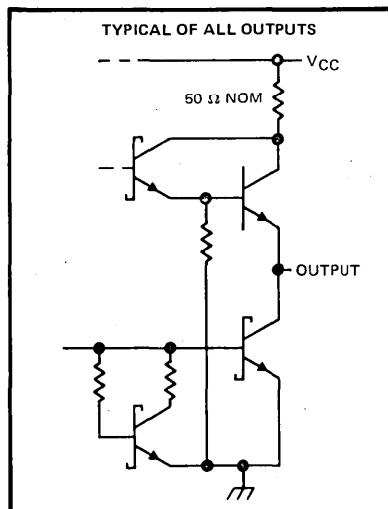
'S113
