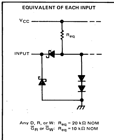
'LS170
