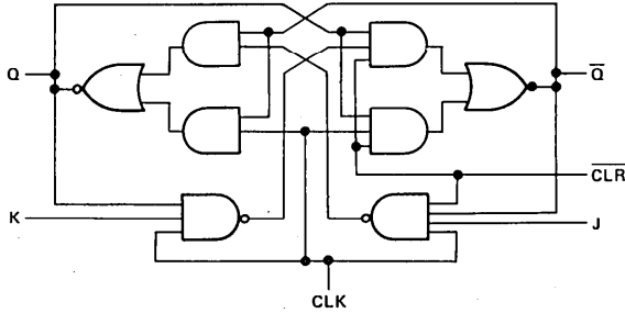
'LS107A
