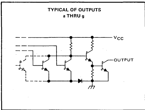
'LS47
