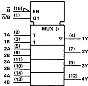
'S257
