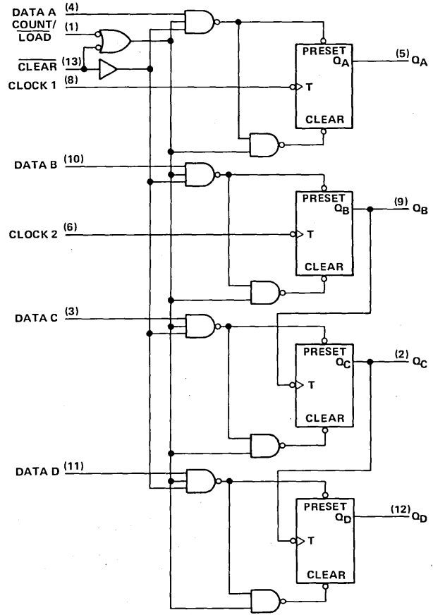
SN54177, SN74177
