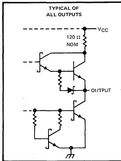
'LS113A
